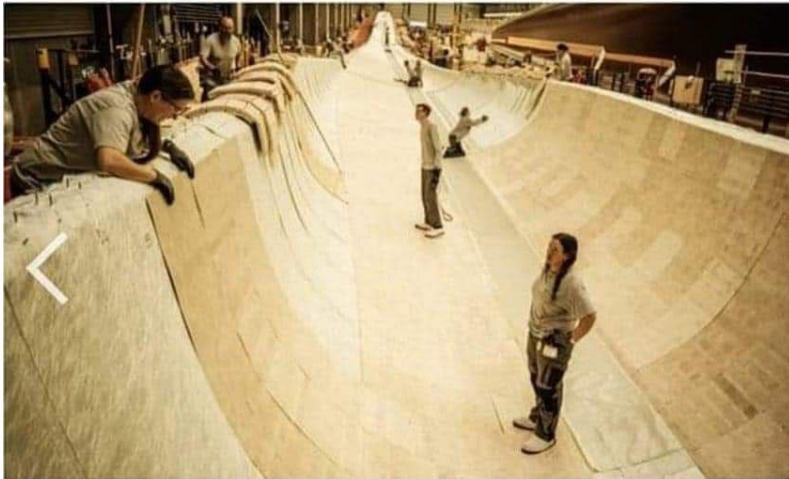
Le balsa sert de matériau de renfort dans une pale de rotor de 81 m de long, ici dans une usine de Siemens-Gamesa au Danemark en février 2022 (© Carsten Snejbjerg)
